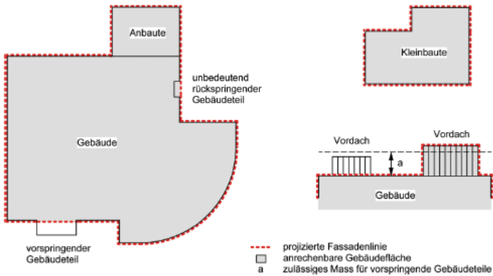
Fig. 8.4 Anrechenbare Gebäudefläche
