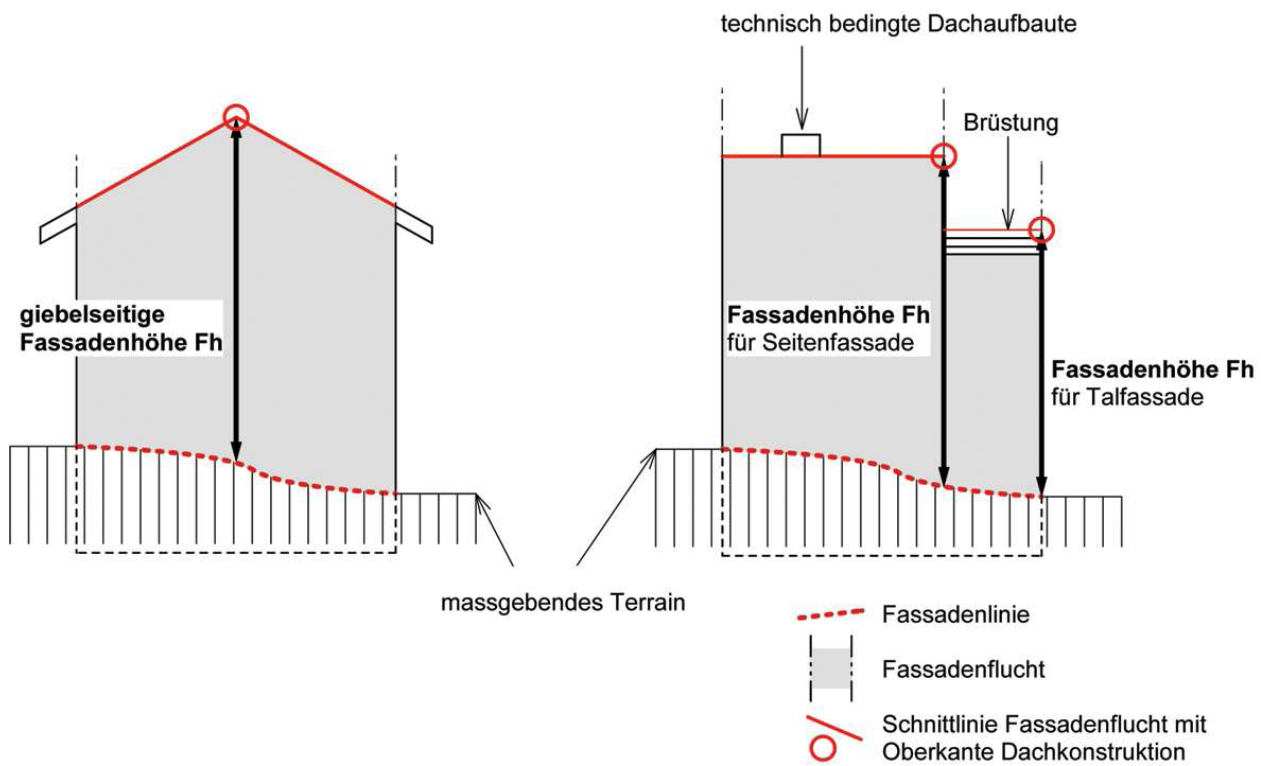
Fig. 5.2 Fassadenhöhe
