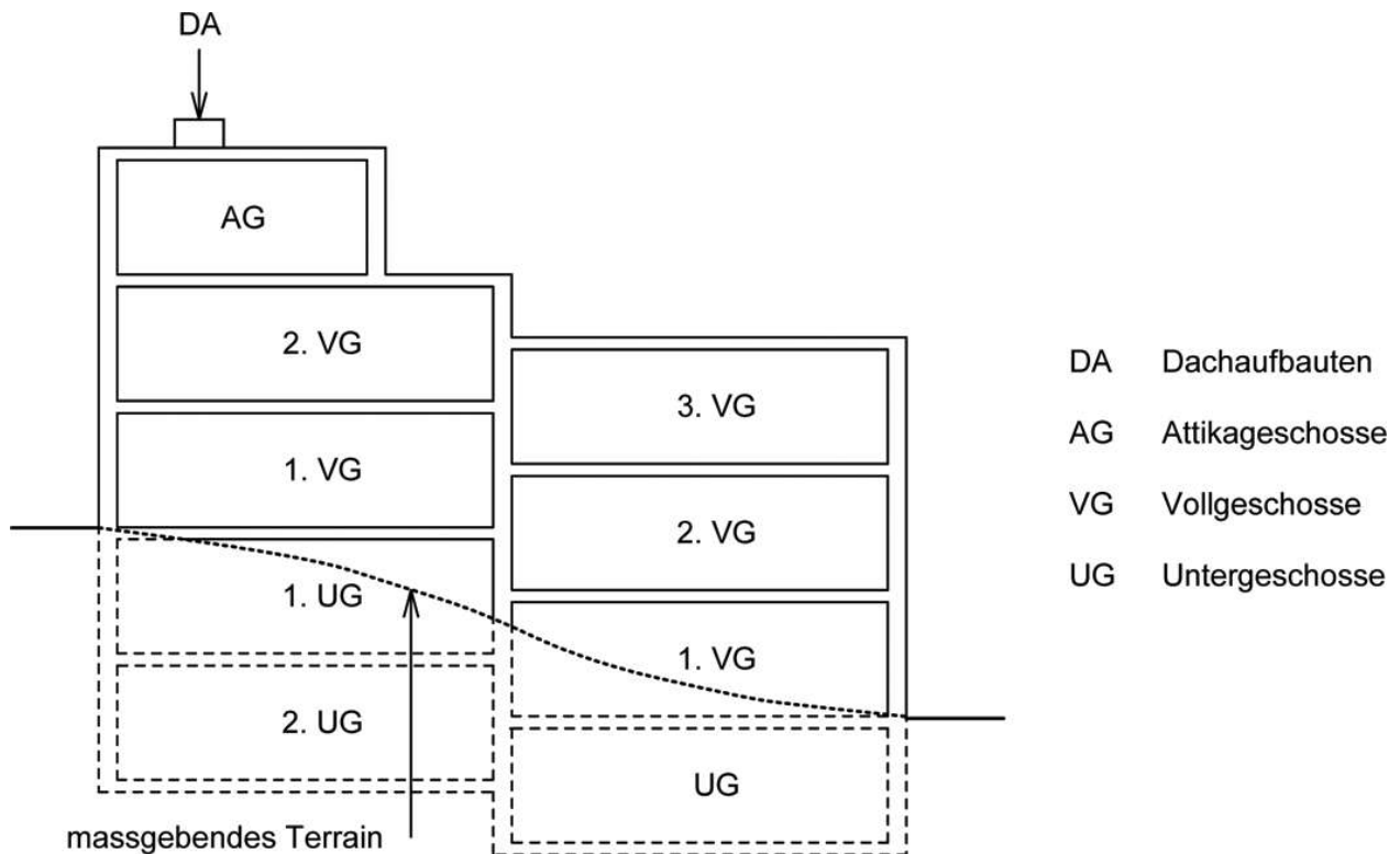
Fig. 6.1 Geschosse und Geschoszahl
