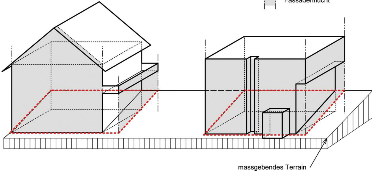
Fig. 3.1 – 3.2 Fassadenflucht und Fassadenlinie
