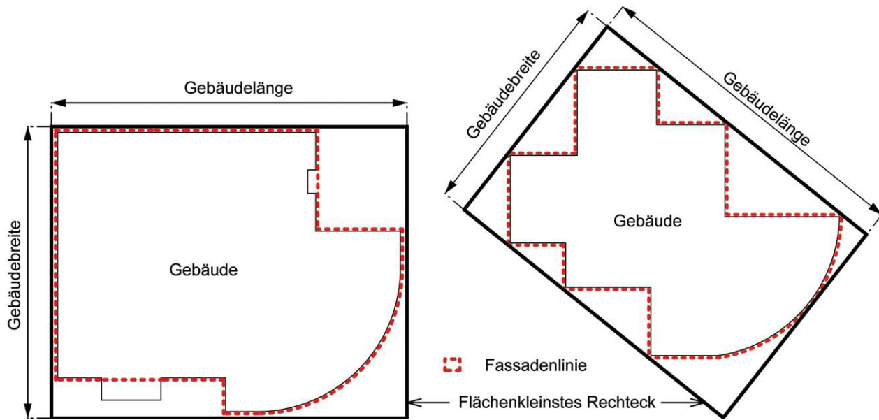
Fig. 4.1 und 4.2 Gebäuelänge und Gebäudebreite
